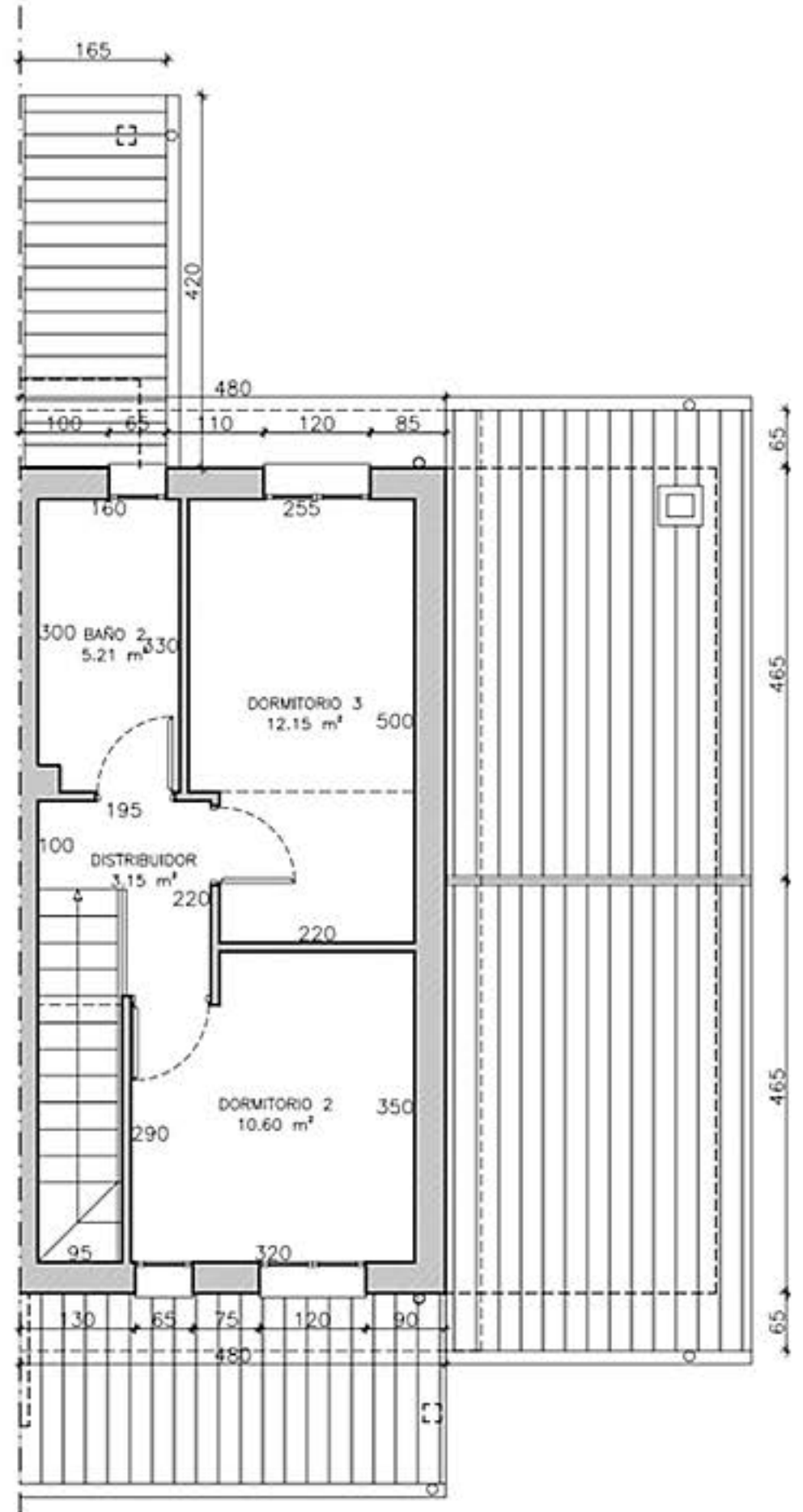
PLANTA PRIMERA
