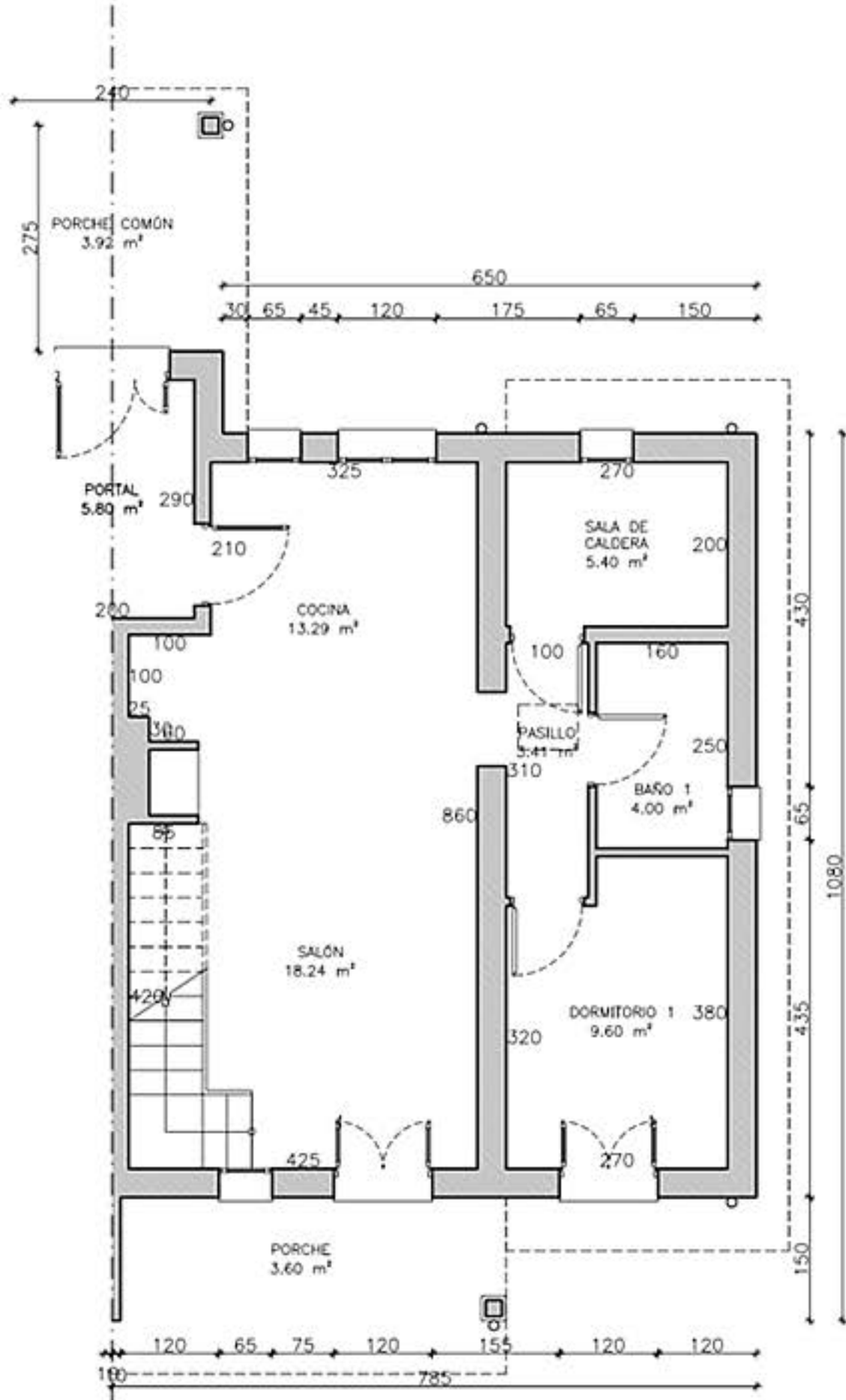
PLANTA BAJA
