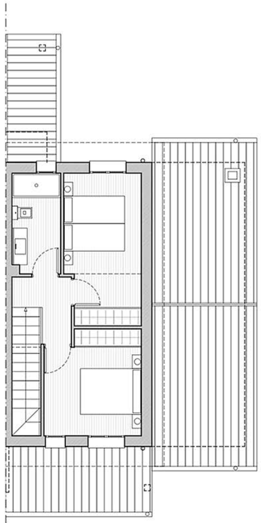
PLANTA PRIMERA
